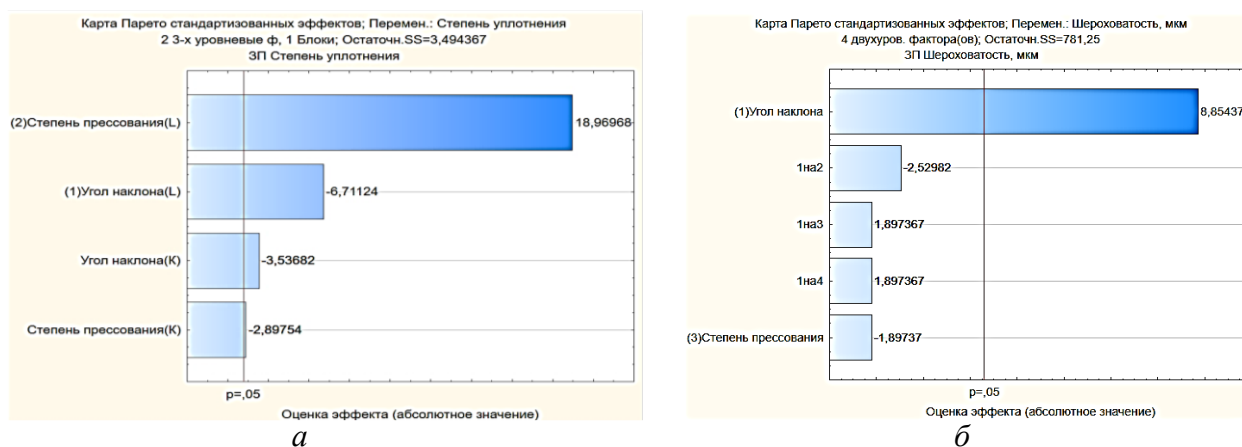
Рисунок 4 – Карта Парето-эффектов для модели отклика: a – твердость лицевой поверхности HRR_l ; б – шероховатость поверхности R_m \max
