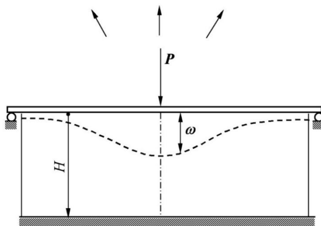
Рис. 2. Расчетная схема пластины на упругом основании
