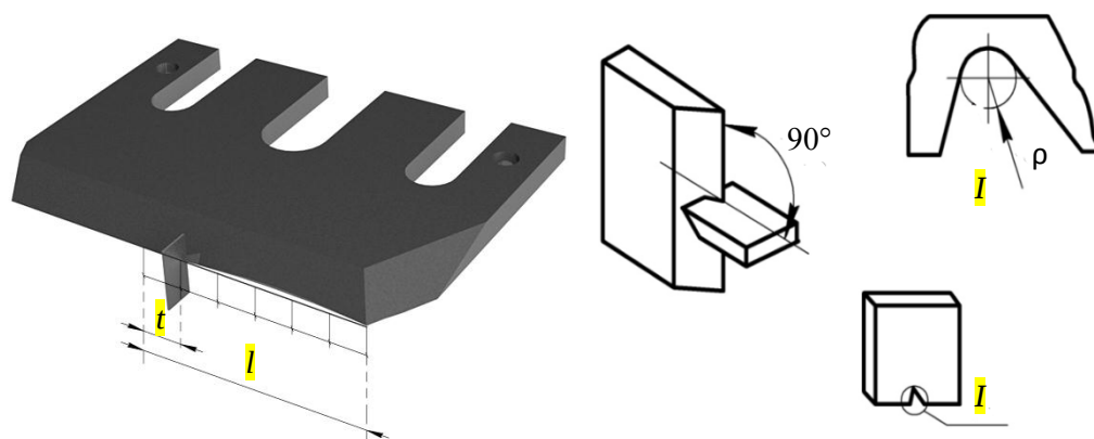
Рис. 5. Метод слепков ( l – выносное изображение)
