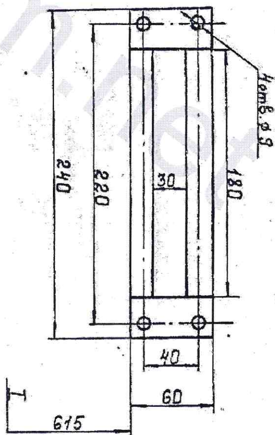
Рис. 8 Схема присоединения станка к вентилятору.
