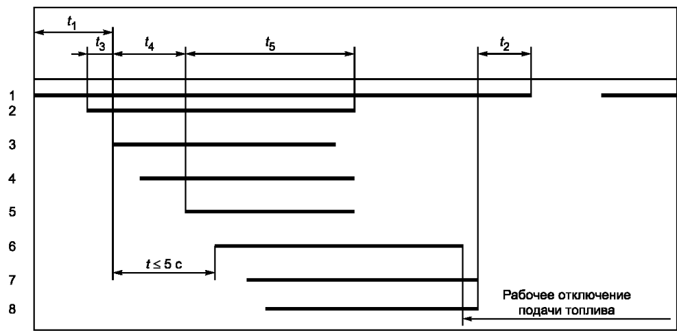
Диаграммы с защитным отключением при пуске
