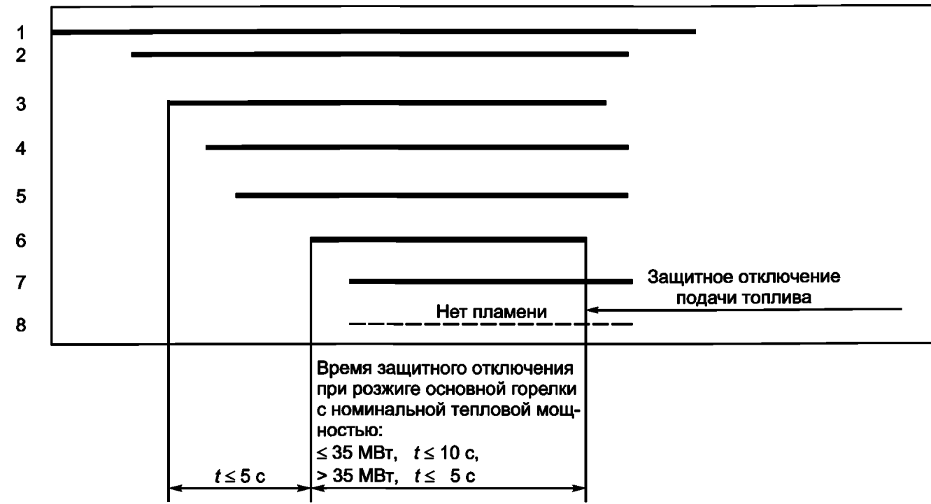
б) Диаграмма работы горелки при погасании пламени основной горелки
