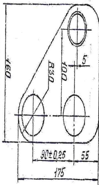
Рис. 6 Кронштейн для пакетов.
