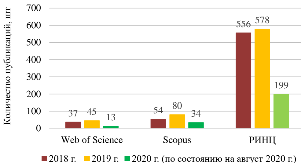
Рис. 1. Диаграмма числа публикаций
