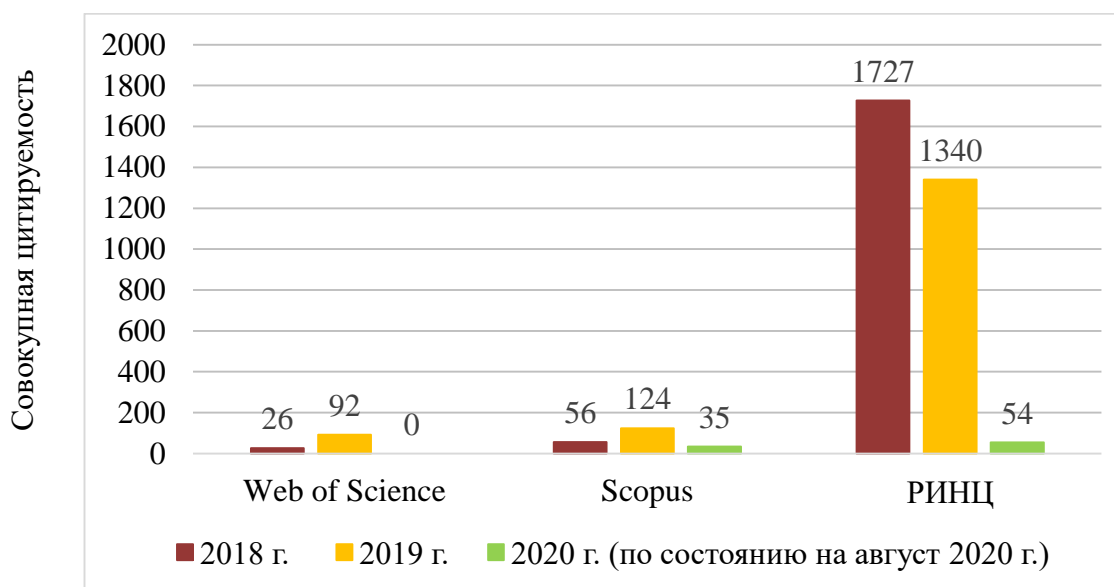
Рис. 2. Диаграмма совокупной цитируемости публикаций
