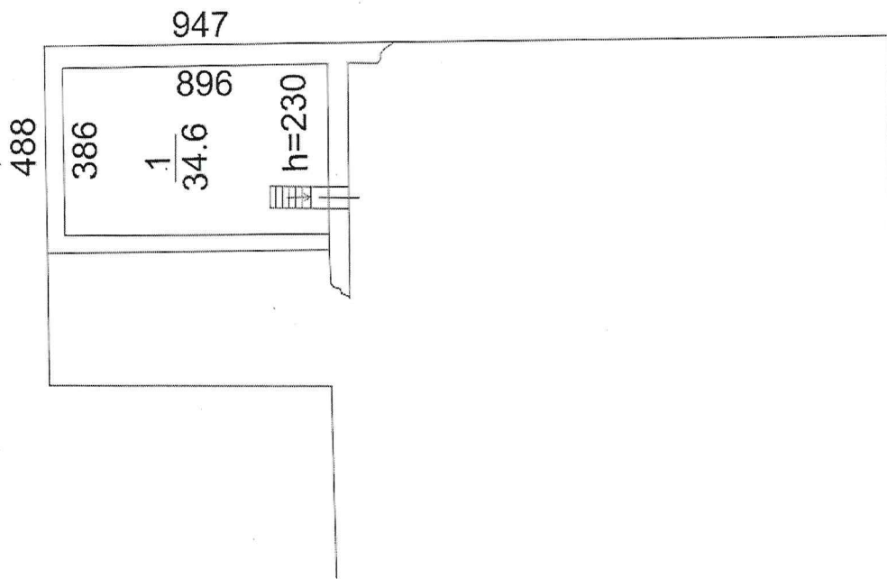
Рис. 1. План подвала
