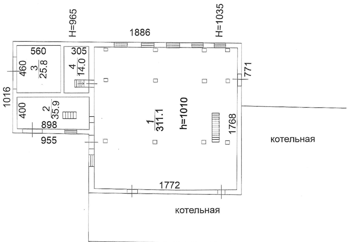
Рис. 2. План 1-го этажа
