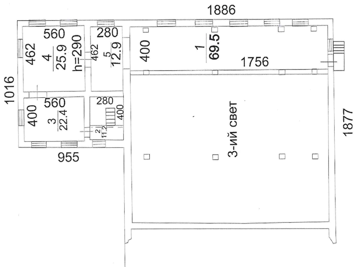
Рис. 4. План 3-го этажа
