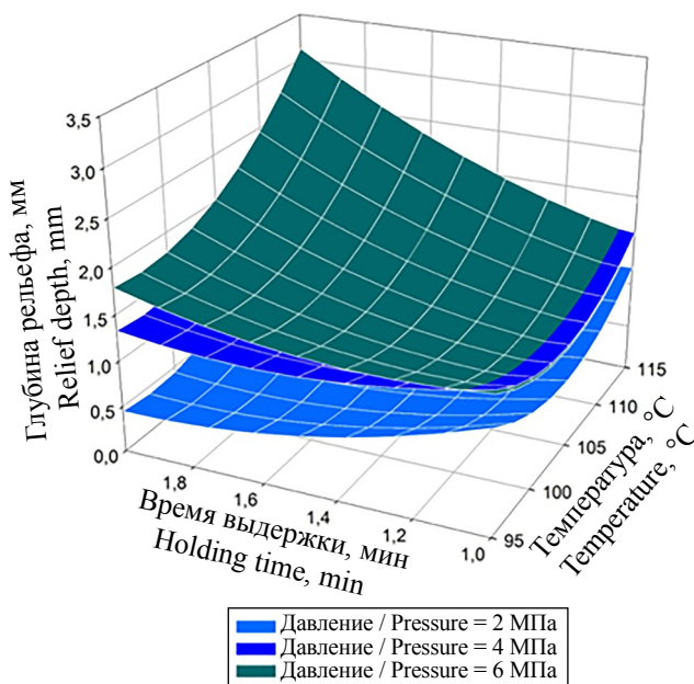
Рис. 3. Влияние параметров режима на глубину рельефа Fig. 3. The effect of the mode parameters on the depth of the relief
