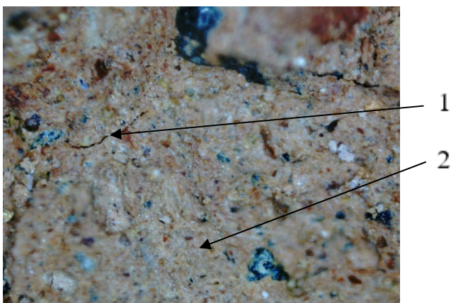
Рисунок 12 – Изображение структуры цементогрунта в возрасте 28 суток твердения: 1 – микротрещина; 2 – цементогрунтовая матрица
