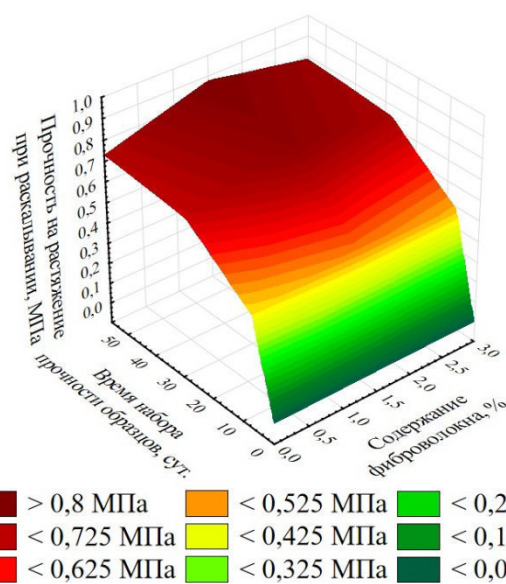
Рисунок 19 – Поверхность отклика прочности на растяжение при раскалывании в зависимости от содержания фиброволокна и времени твердения
