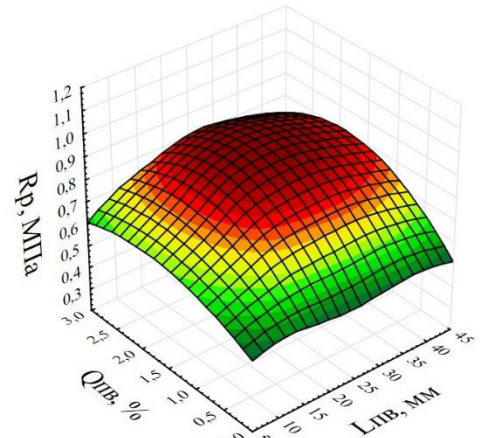
Рисунок 6 – Поверхность отклика прочности на растяжение при раскалывании в зависимости от длины и содержания полипропиленового волокна
