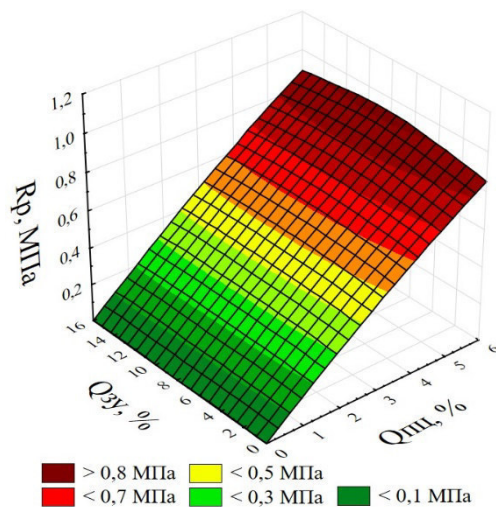
Рисунок 25 – Поверхность отклика прочности на растяжение при раскалывании в зависимости от содержания портландцемента и золы-уноса ГРЭС
