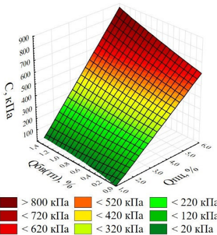
Рисунок 8 – Поверхность отклика удельного сцепления в зависимости от содержания портландцемента и фиброволокна
