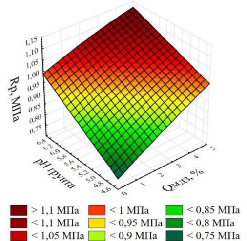
Рисунок 23 – Поверхность отклика прочности на растяжение при раскалывании в зависимости от содержания минеральной добавки на основе золы-уноса ГРЭС и кислотности грунта (pH)
