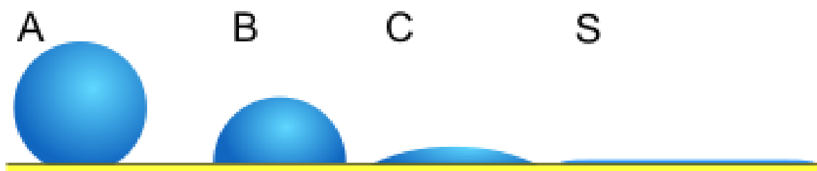
Рис. 1. Варианты смачивания:
