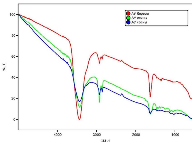
Рисунок 10 – ИК-спектры образцов активных углей, полученных при температуре пиролиза 800 °С, температуре активации 900 °С, удельный расход пара – 1,8 кг/кг древесного угля, продолжительность процесса активации – 100 мин
