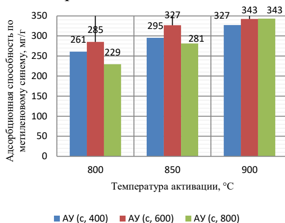
Рисунок 6 – Зависимость влияния температуры активации на адсорбционную активность по метиленовому синему для АУ, полученных из сосновых ДУ при разных температурах пиролиза
