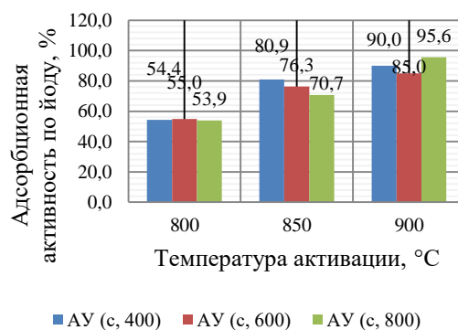
Рисунок 5 – Зависимость влияния температуры активации на адсорбционную активность по йоду для активных углей, полученных из сосновых ДУ при разных температурах пиролиза
