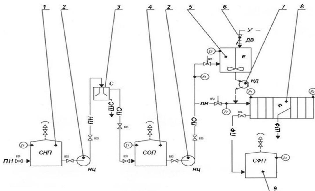
Рисунок 14 – Схема обработки нефilterованного пива активным осиновым углем
