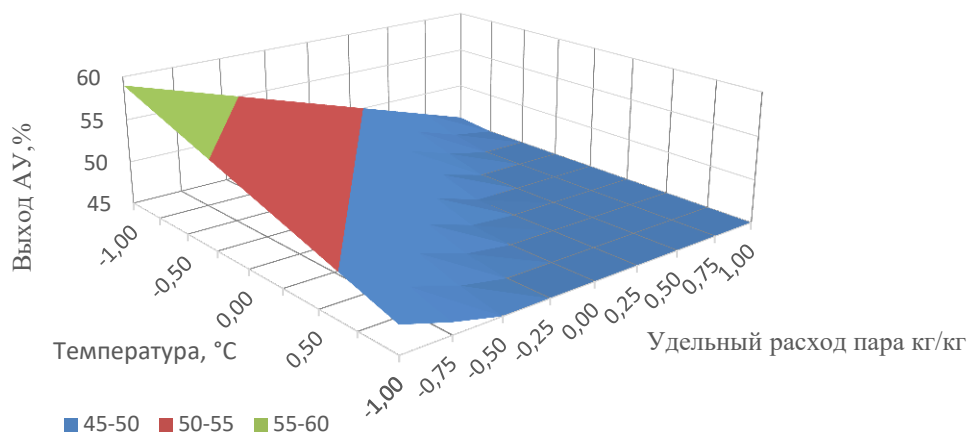
Рисунок 7 – Зависимость выхода осинового активного угля от температуры активации и удельного расхода пара
