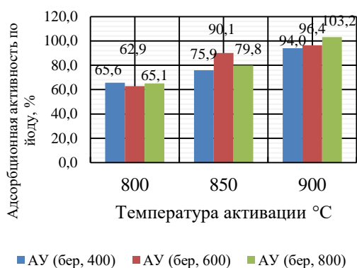
Рисунок 1 – Зависимость влияния температуры активации на адсорбционную активность по йоду для АУ, полученных из березовых ДУ при разных температурах пиролиза
