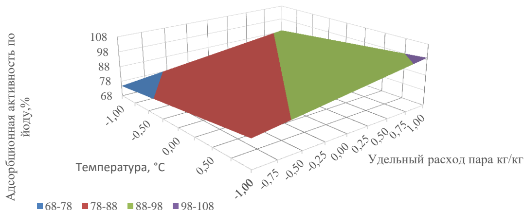
Рисунок 8 – Зависимость адсорбционной активности по йоду осинового АУ от температуры активации и удельного расхода пара
