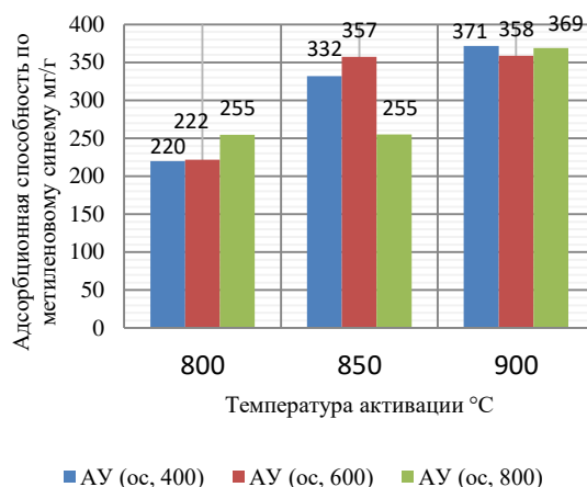
Рисунок 4 – Зависимость влияния температуры активации на адсорбционную активность по метиленовому синему для АУ, полученных из осиновых ДУ при разных температурах пиролиза
