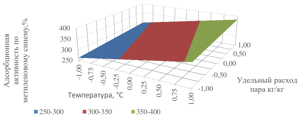
Рисунок 9 – Зависимость адсорбционной активности по метиленовому синему АУ осины от температуры активации и удельного расхода пара
