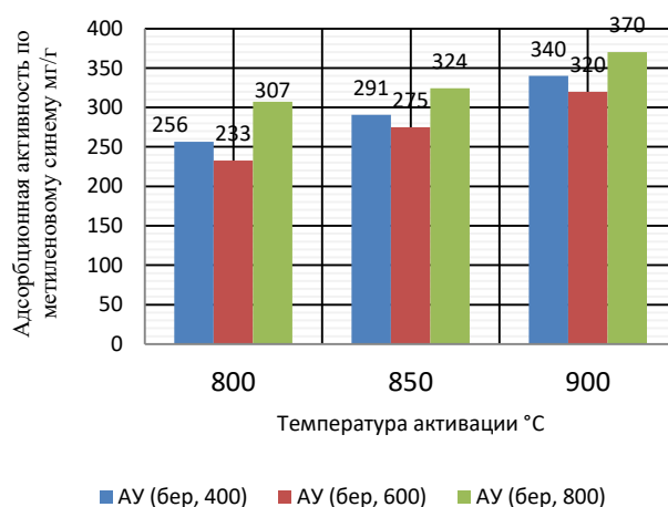
Рисунок 2 – Зависимость влияния температуры активации на адсорбционную активность по метиленовому синему для АУ, полученных из березовых ДУ при разных температурах пиролиза
