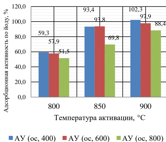
Рисунок 3 – Зависимость влияния температуры активации на адсорбционную активность по йоду АУ, полученных из осиновых ДУ при разных температурах пиролиза
