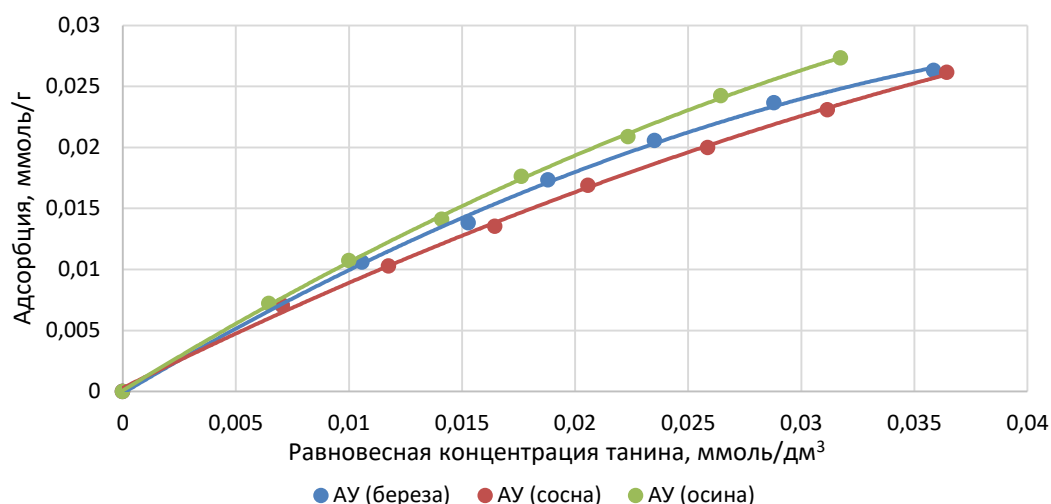
Рисунок 11 – Изотермы сорбции танина экспериментальными углями
