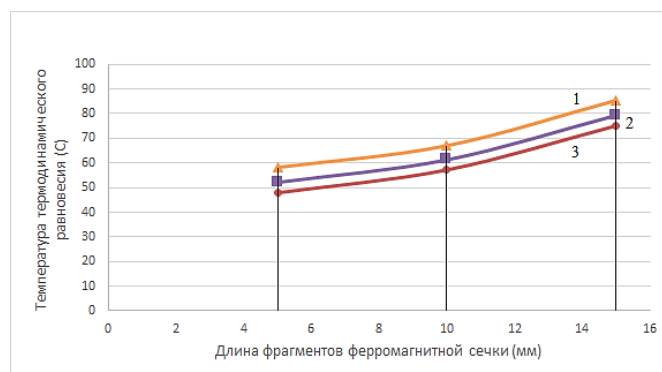
Рис. 7. Индукционный нагрев ферромагнитной сечки из стальной проволоки током частотой f = 7,3 кГц 1 – фракции 1230 мкм; 2 – фракции 380 мкм; 3 – фракции 330 мкм
