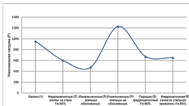
Рис. 9. Прочность клеевого соединения с наполнителями на основе эпоксидной клеевой композиции
