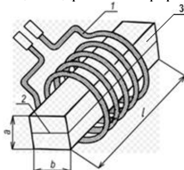
Рис. 1 Пространственная модель нагрева клеевого шва с ферромагнитным наполнителем цилиндрическим индуктором: 1 – индуктор; 2 – клеевой шов; 3 – древесина l – длина; b – ширина; a – высота
