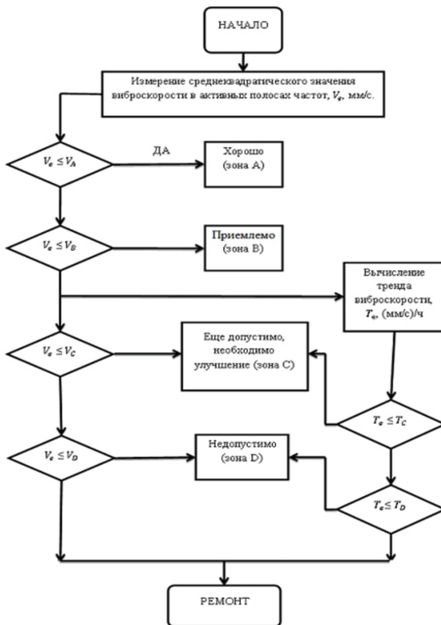
Блок-схема алгоритма определения технического состояния оборудования ЦБП Block diagram of the algorithm for determining the technical condition of the CVP equipment
